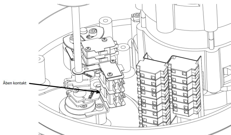
Figur 2: Åben kontakt
