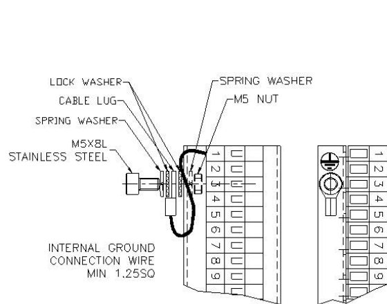
Indvendig jordforbindelse
