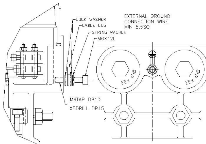
Udvendig jordforbindelse
